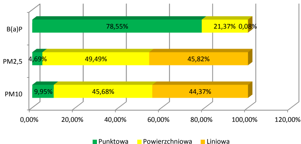
Rysunek 48. Procentowe udziały poszczególnych źródeł emisji w rocznej emisji pyłu zawieszanego PM10, PM2,5 oraz benzo(a)pirenu w Rzeszowskim Obszarze Funkcjonalnym w 2013 roku 118
