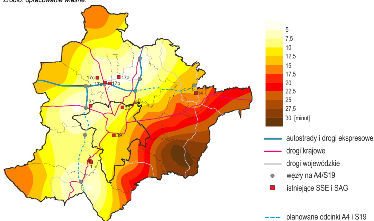
Rys. 35. Czas dojazdu samochodem do węzłów na drodze ekspresowej S19 po realizacji brakującego odcinka A4 i brakujących odcinków S19 w Rzeszowskim Obszarze Funkcjonalnym na tle istniejących SAG.
