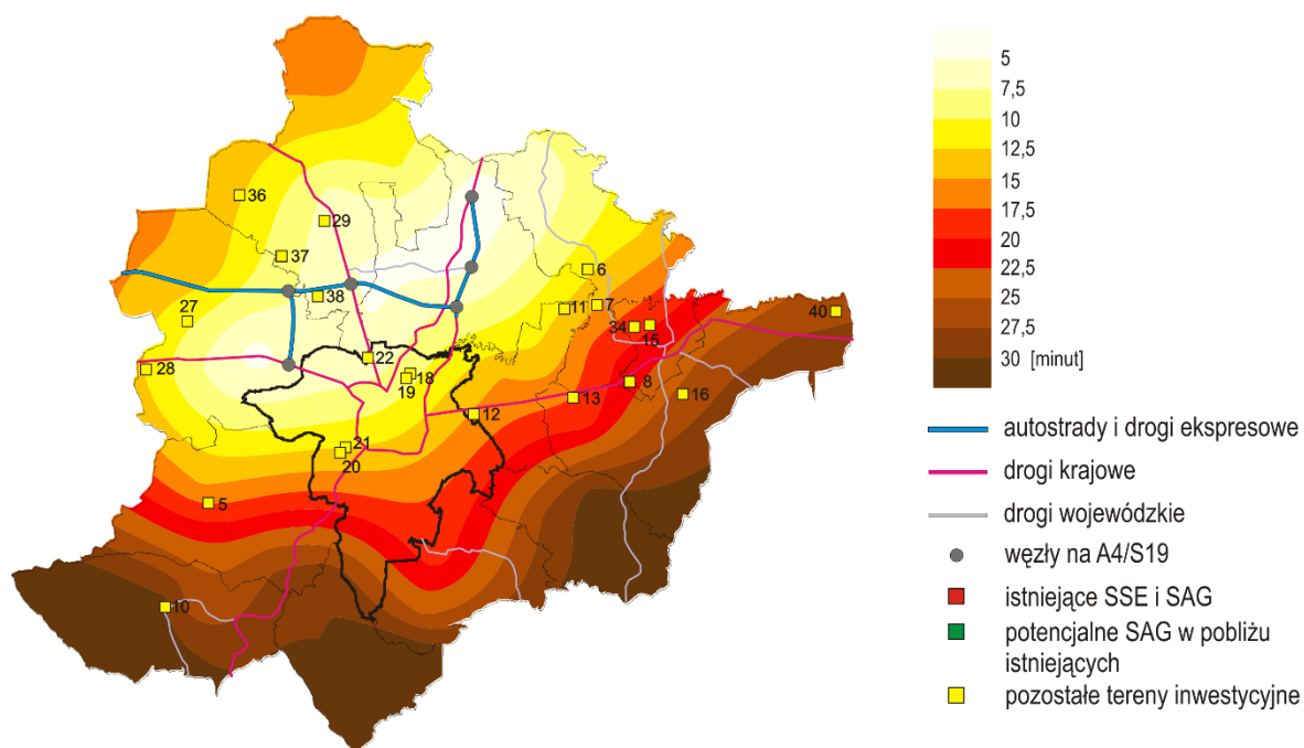
Rys. 45. Czas dojazdu samochodem do węzłów na drodze ekspresowej S19 w Rzeszowskim Obszarze Funkcjonalnym w 2014 r. na tle pozostałych terenów inwestycyjnych w 2014 r.
