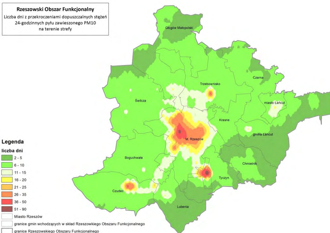
Rysunek 62. Rozkład liczby dni z przekroczeniem dopuszczalnej wartości stężenia 24-godzinne dla pyłu zawieszonego PM10 w Rzeszowskim Obszarze Funkcjonalnym w roku bazowym 2013 273
